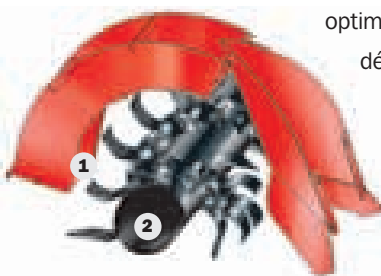
Grande performance: le rotor de grande dimension (2) silencieux et robuste. Les contre-couteaux (1) procurent une coupe soignée.
