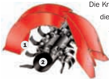
Starke Leistung: Die großdimensionierte Schlegelwelle (2) überzeugt durch Lauf-ruhe und Stabilität. Die Gegenschneide (1) sorgt für ein sauberes Schnittbild.
